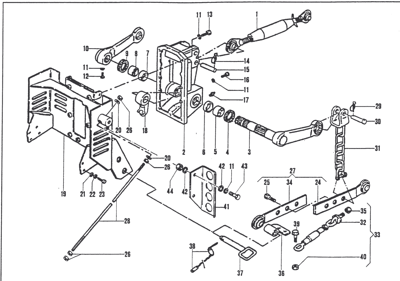
ATTACCO A TRE PUNTI CON PORTATTREZZI ANTERIORE - THREE POINT HITCH LINKAGE WITH FRONT LIFTER - ATTELAGE A TROIS POINTS AVEC RELEVAGE AVANT - DREIPUNKT ANSCHLUSS MIT VORDEREN KRAFTHEBER - ENGANCHE EN 3 PUNTOS CON ELEVADOR DELANTERO
