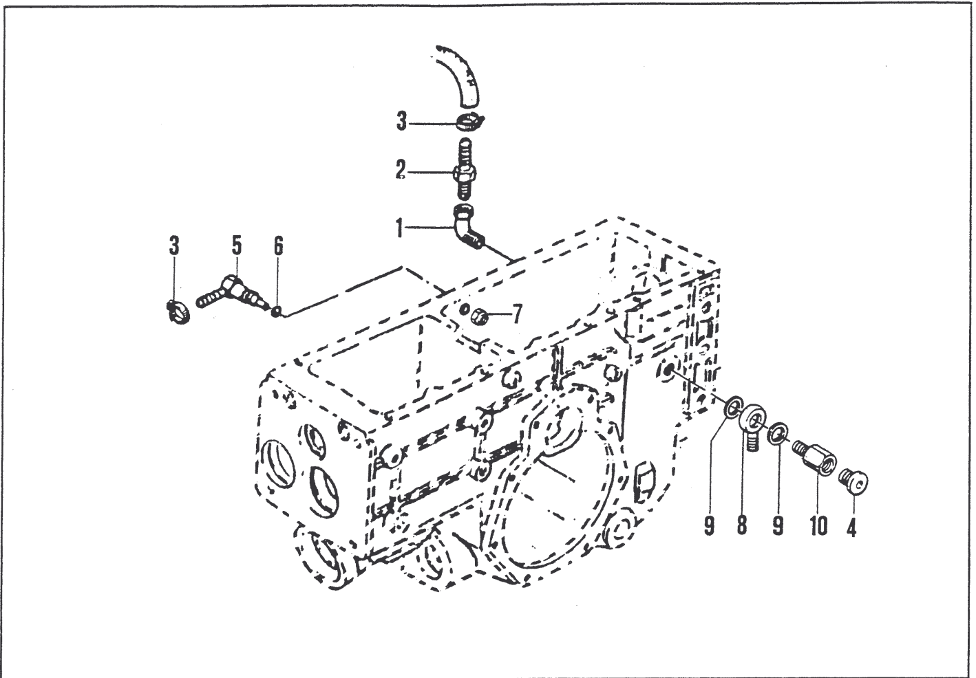
COLLEGAMENTI IDRAULICI SCATOLA CAMBIO E DEVIATORE - HYDRAULIC CONNECTIONS FOR GEARBOX - CONNEXIONS HYDRAULIQUES BOITE DE VITESSES - HYDRAULISCHE ANSCHLUESSE SCHALTGETRIEBE - CONEXIONES HYDRAULICAS CAJA DEL CAMBIO
